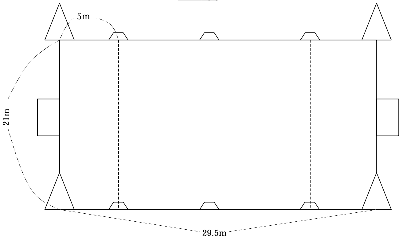
コート図
